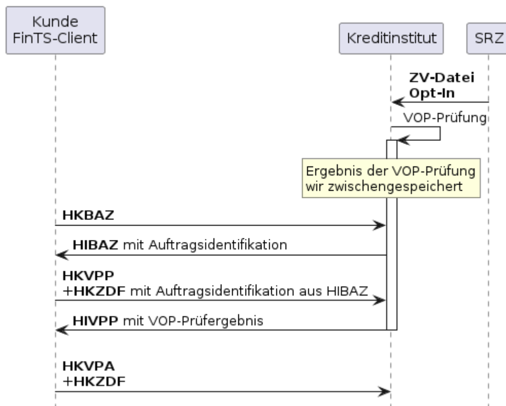
Abbildung 12: Ablauf bei Einreichung durch das SRZ als Opt-In 1
