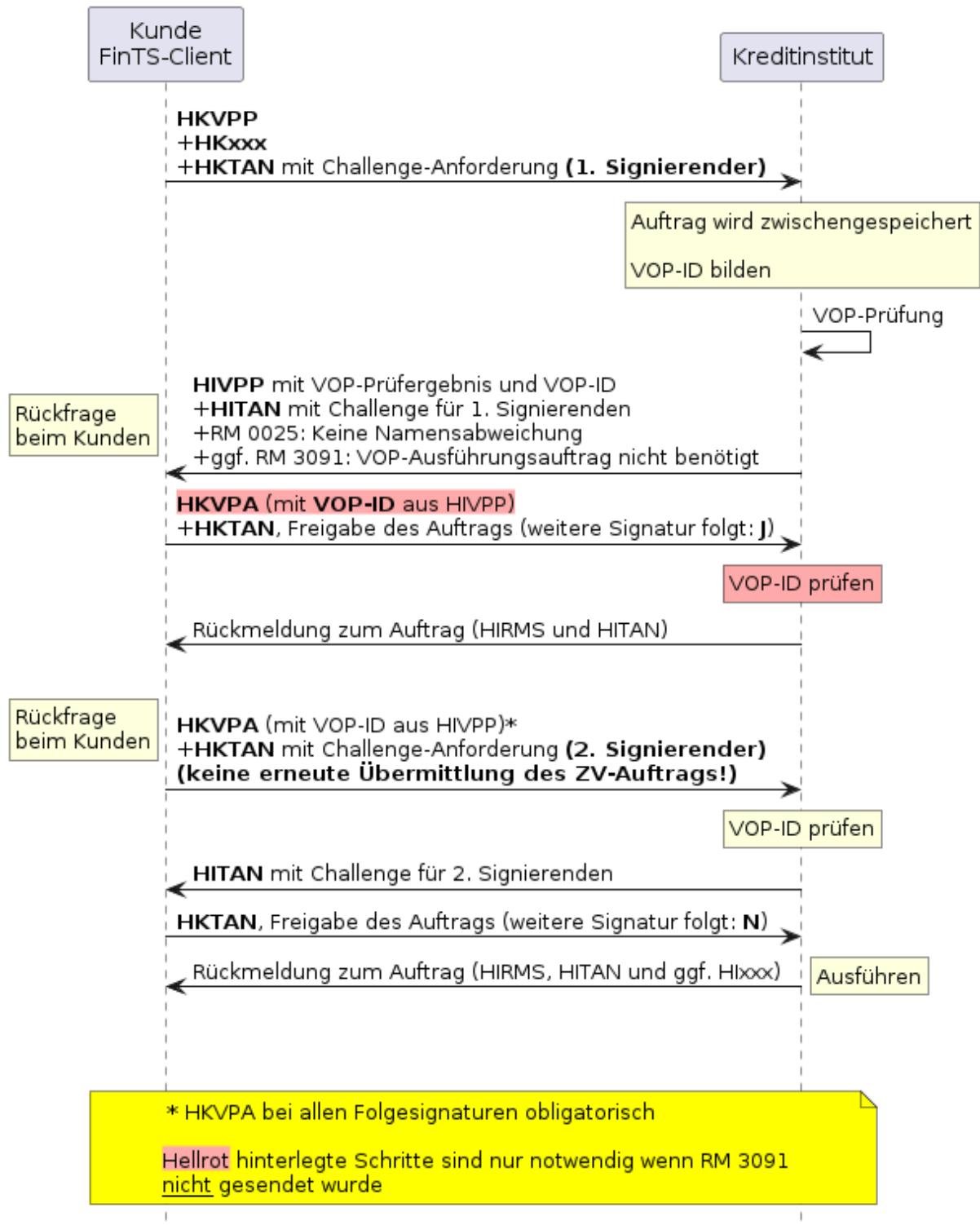
Abbildung 6: Ablauf Namensabgleich VOP mit Mehrfachsignatur und Match in einem Dialog
