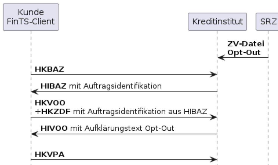
Abbildung 16: Ablauf bei Einreichung durch das SRZ als Opt-Out, Kundenwunsch bei Freigabe: Opt-Out 5
