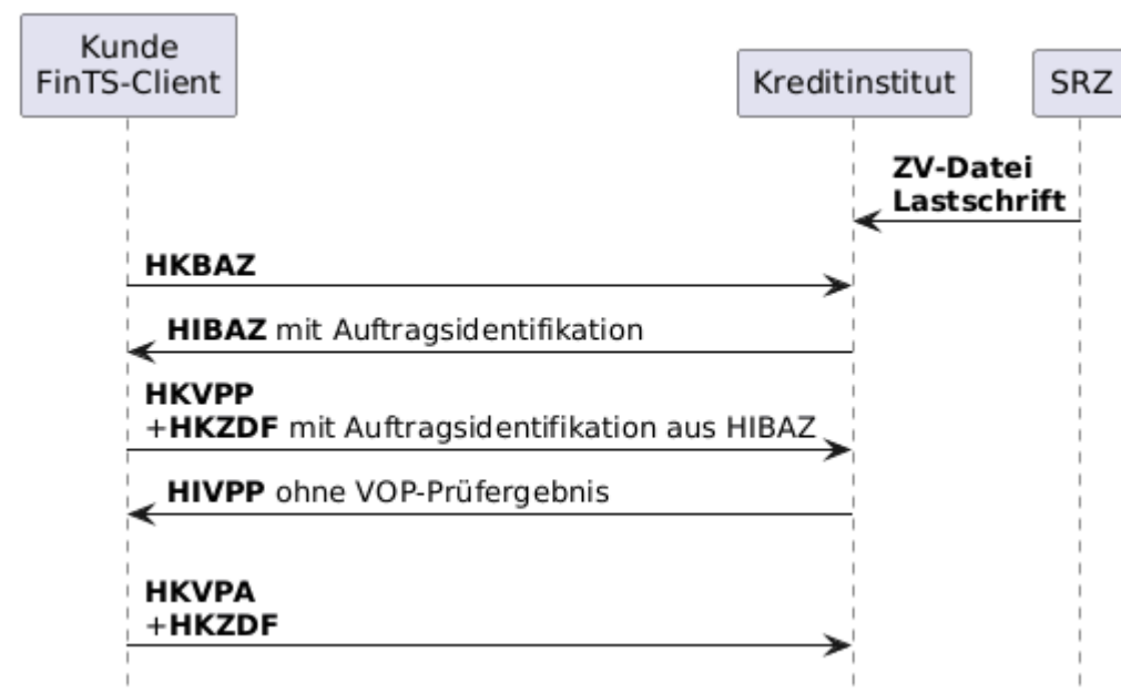
Abbildung 18: Ablauf bei Einreichung von Lastschriften durch das SRZ 7
