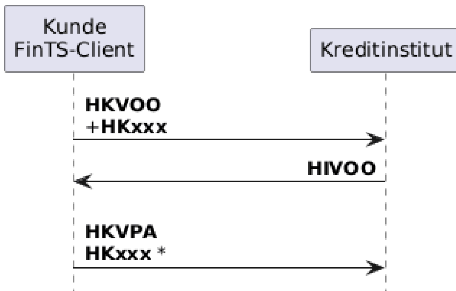
Abbildung 2: Grobskizze des Ablauf ohne Namensabgleich mit HKVOO bei Opt-Out (ohne detaillierte Berücksichtigung eines Sicherheitsverfahrens)*
