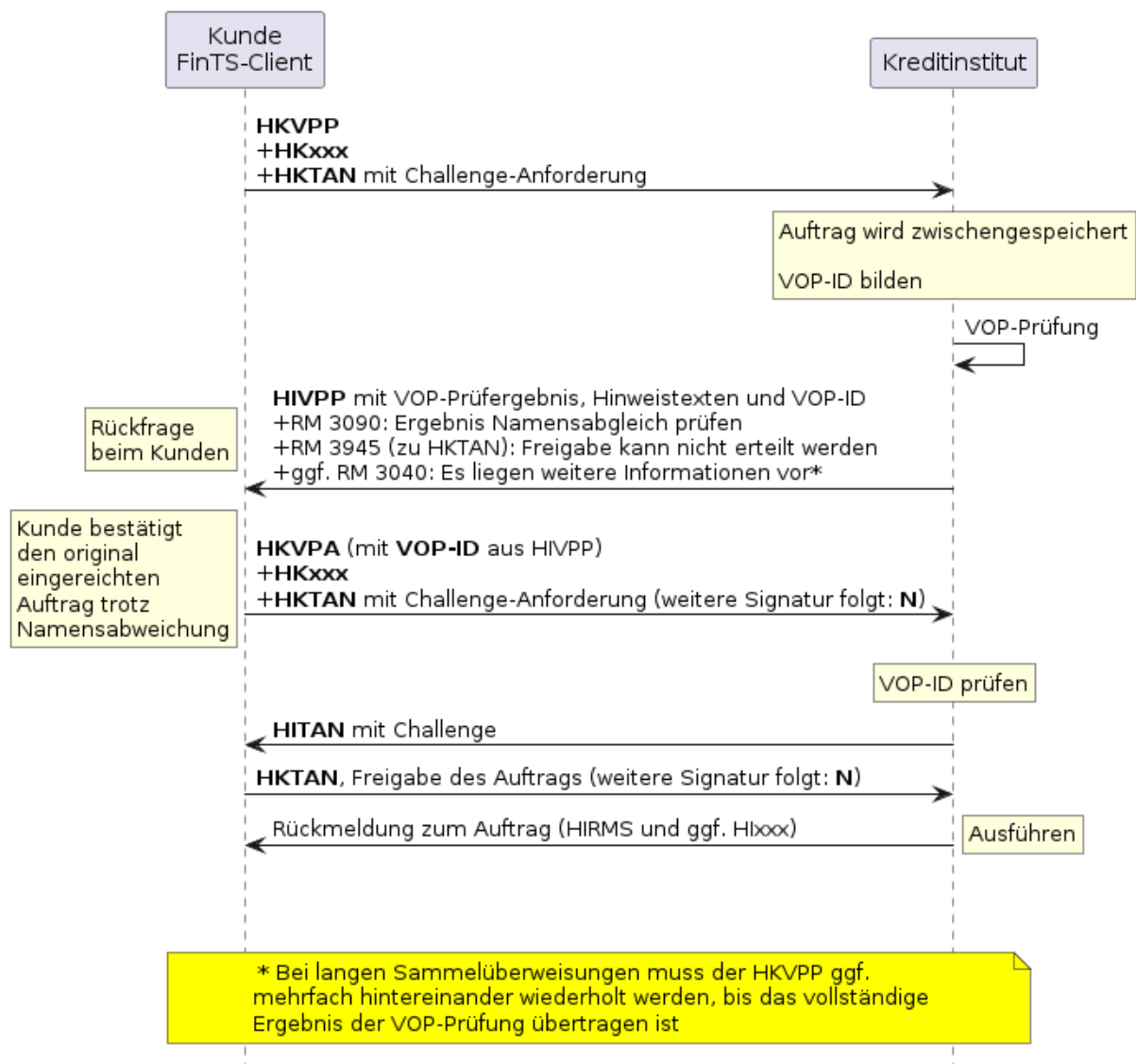
Abbildung 4: Ablauf Namensabgleich VOP mit Einzelsignatur und Close-/No-Match bzw. Not Applicable
