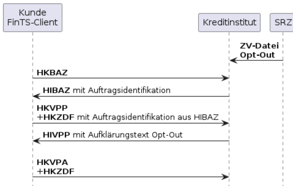
Abbildung 13: Ablauf bei Einreichung durch das SRZ als Opt-Out 2
