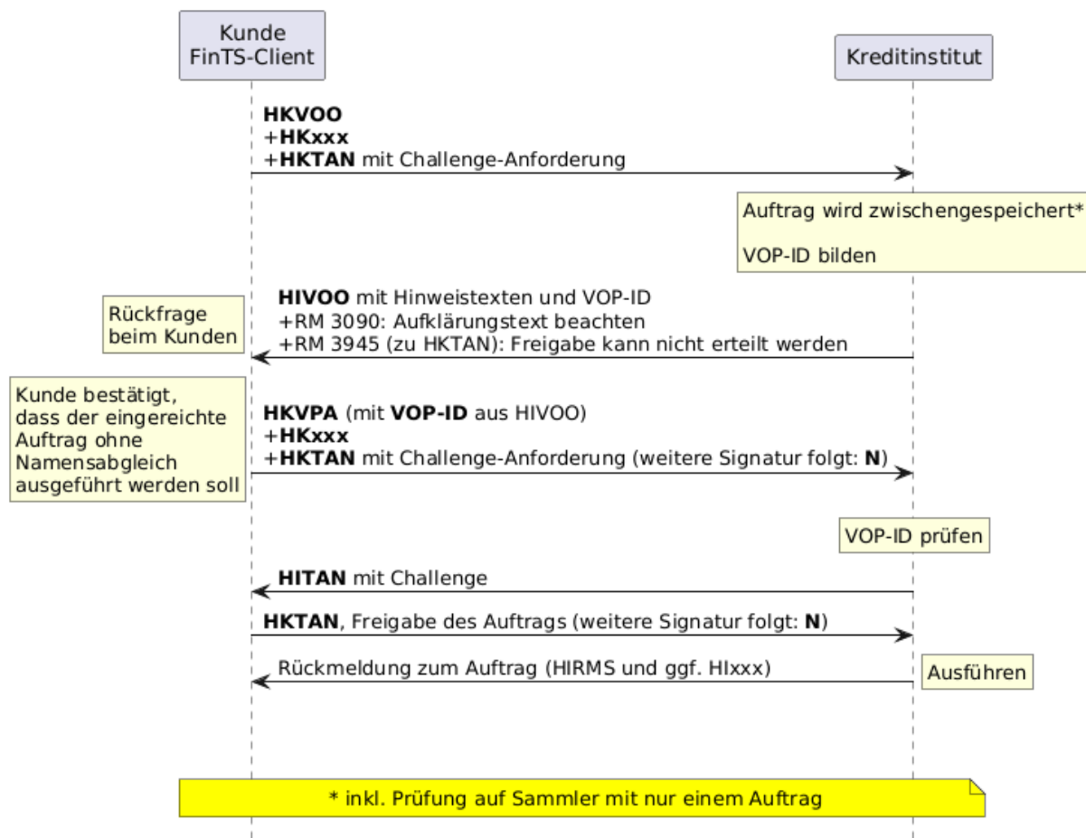
Abbildung 5: Ablauf Opt-Out mit Einfachsignatur
