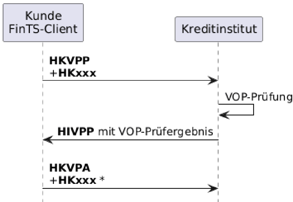
Abbildung 1 Grobskizze des Ablaufs und Zusammenspiels von HKVPP und HKVPA bei Opt-In (ohne detaillierte Berücksichtigung eines Sicherheitsverfahrens)*
