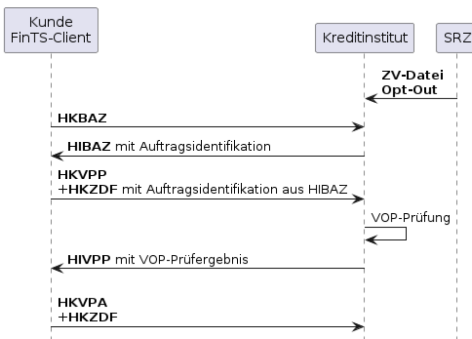
Abbildung 17: Ablauf bei Einreichung durch das SRZ als Opt-Out, Kundenwunsch bei Freigabe: Opt-In 6
