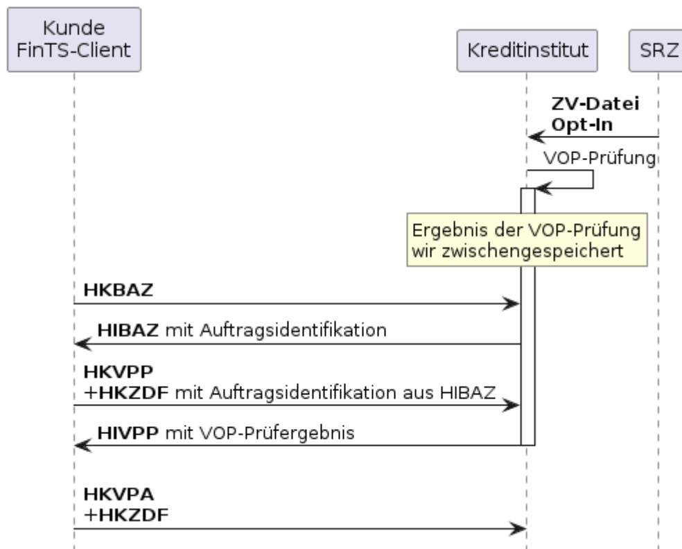
Abbildung 14 Ablauf bei Einreichung durch das SRZ als Opt-In, Kundenwunsch bei Freigabe: Opt-In 3
