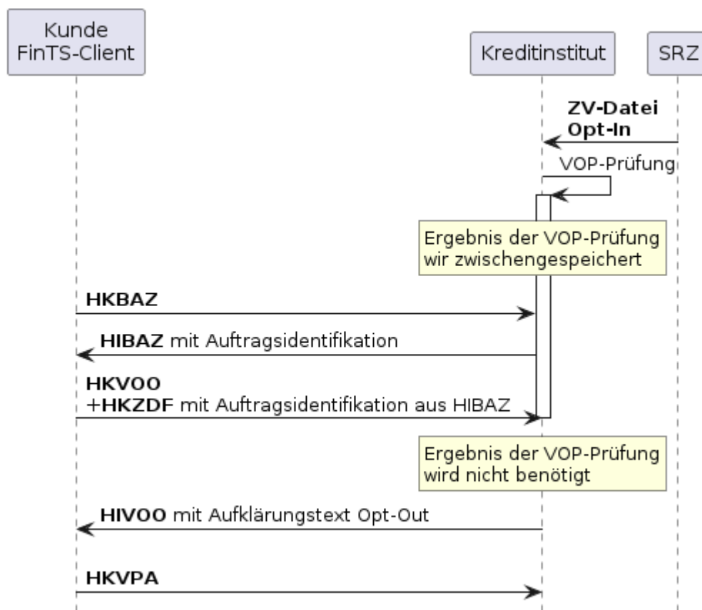
Abbildung 15: Ablauf bei Einreichung durch das SRZ als Opt-In, Kundenwunsch bei Freigabe: Opt-Out 4
