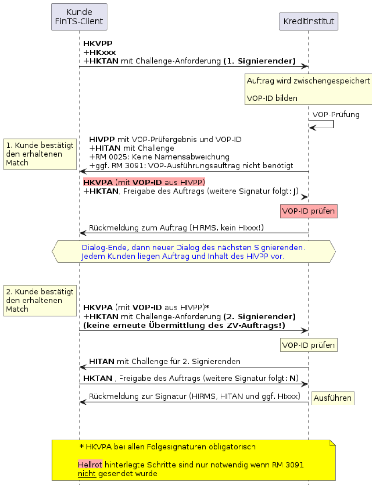
Abbildung 8: Ablauf Namensabgleich VOP mit Mehrfachsignatur und Match in mehreren Dialogen
